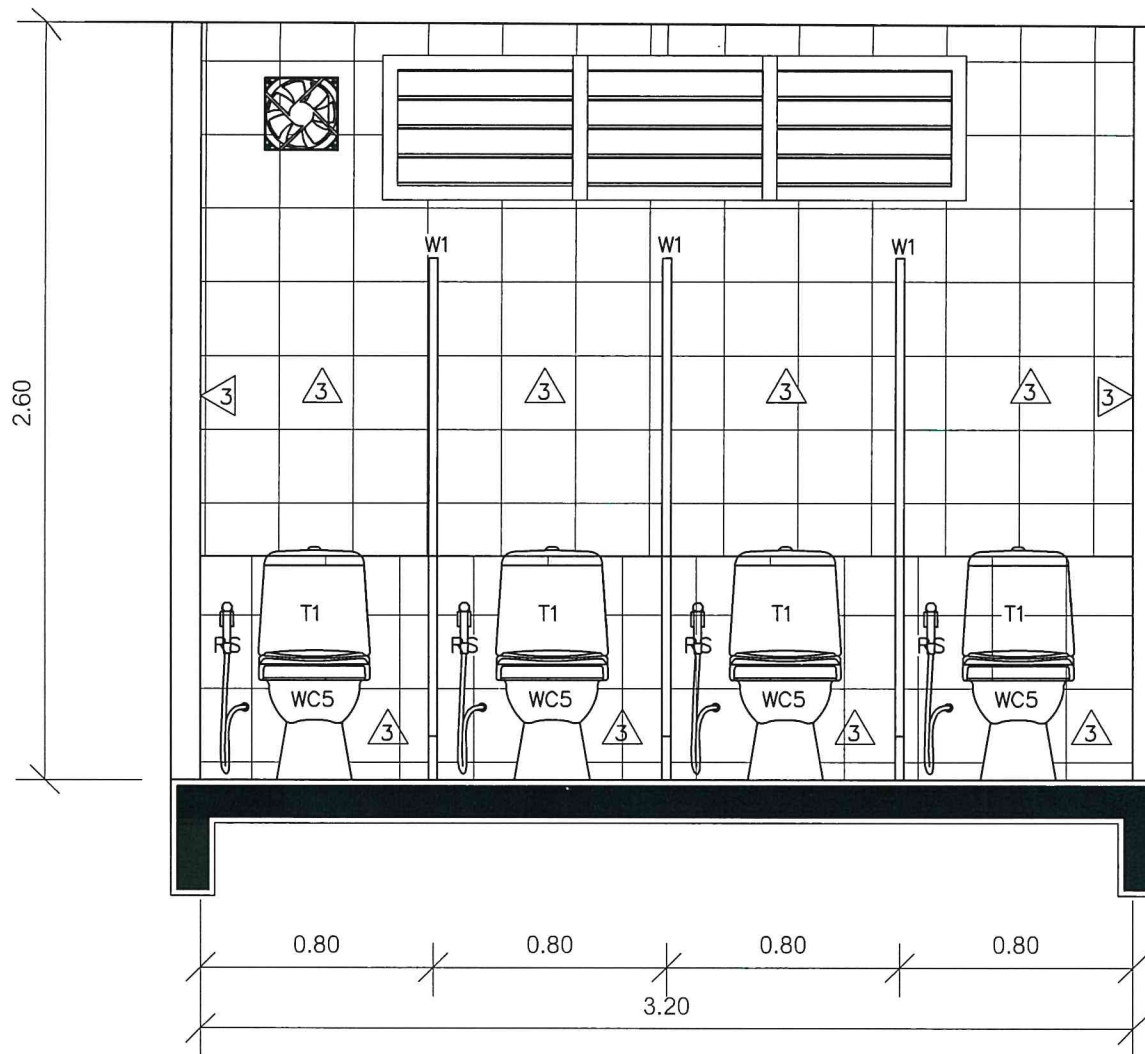
รูปตัด B
