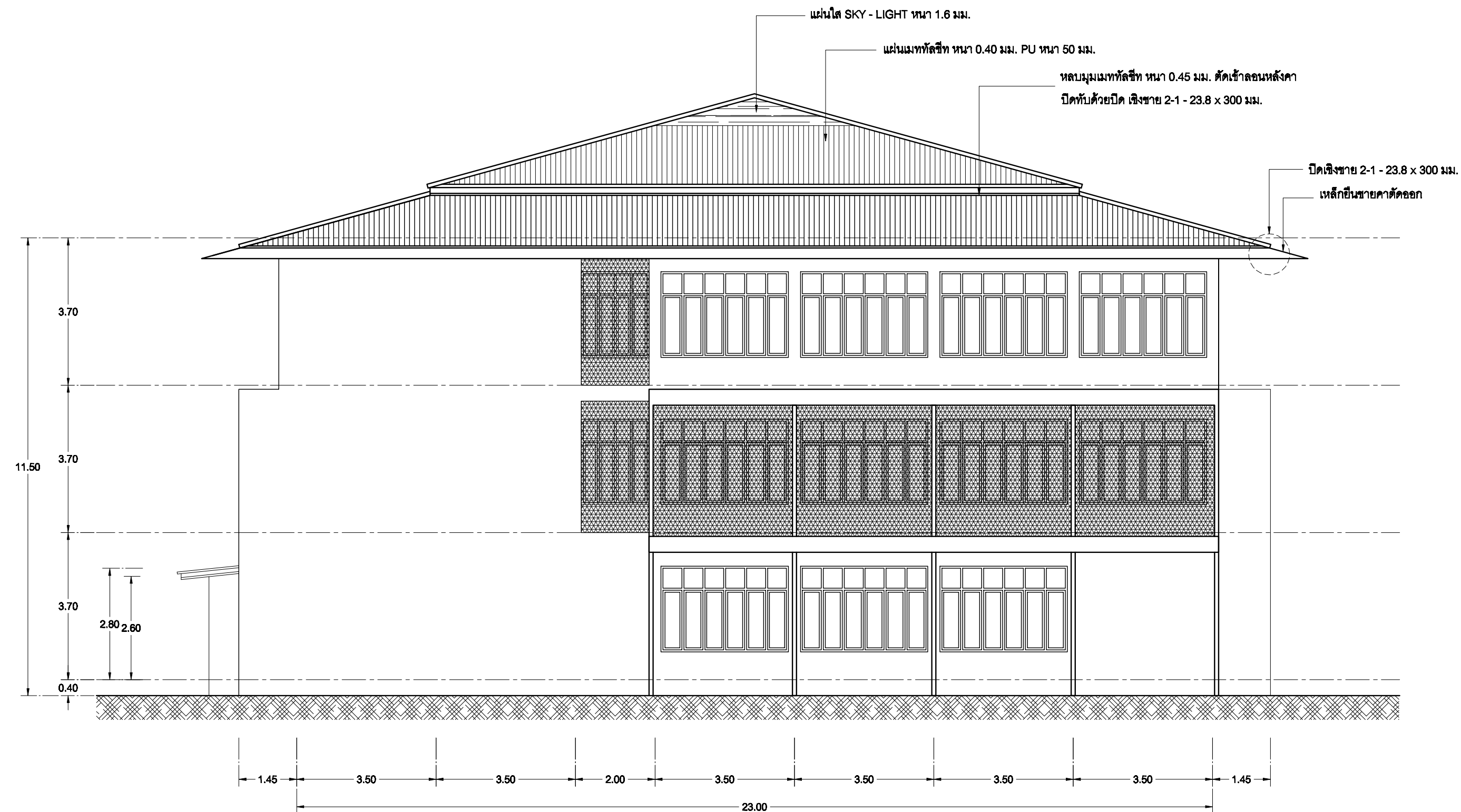
แบบรูปด้าน 3 มาตราส่วน 1 : 100
