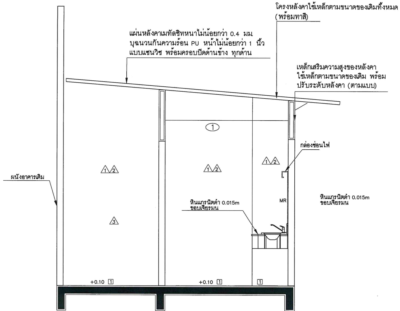
รูปตัด B
