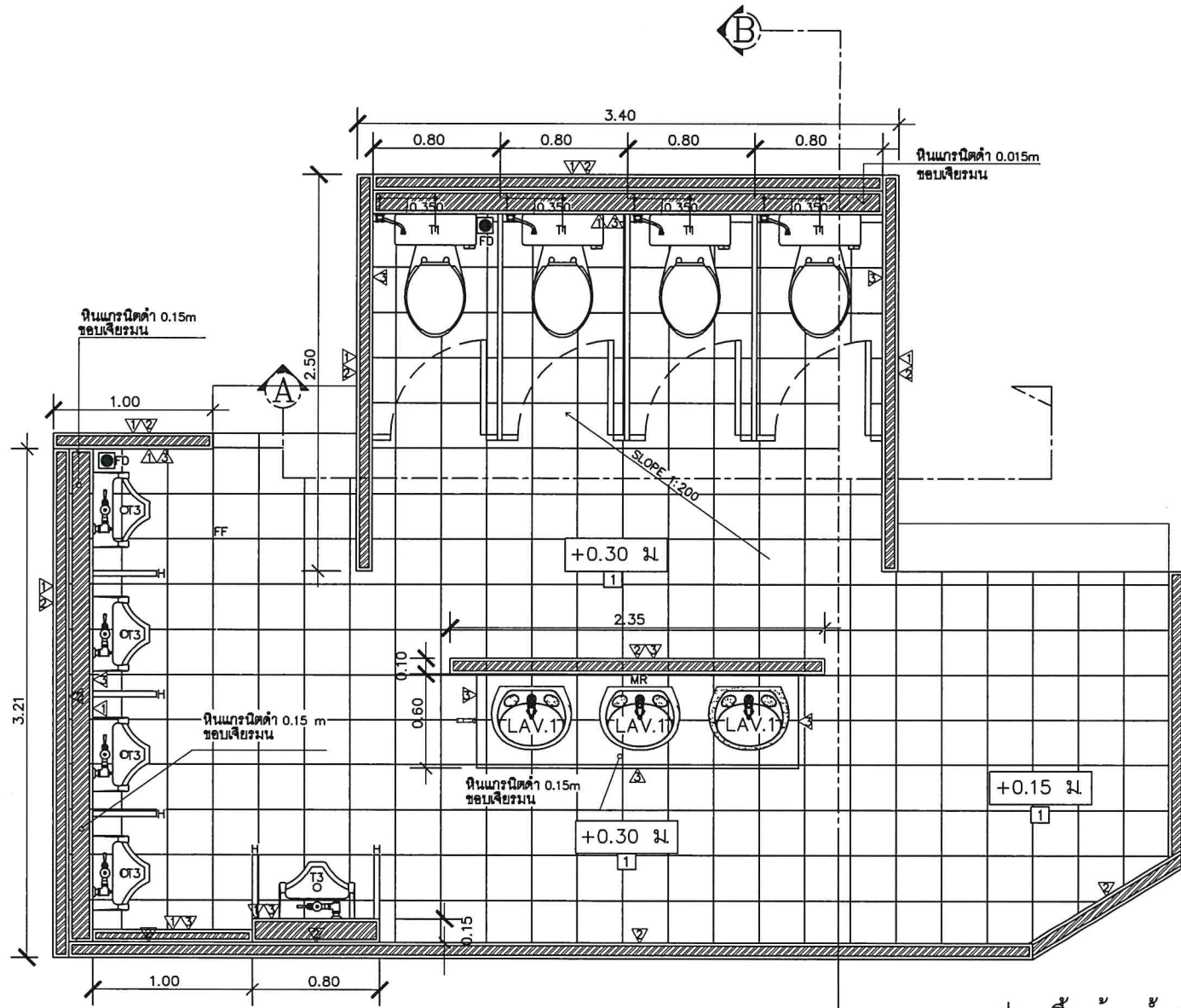
แปลนพื้นห้องน้ำชาย
