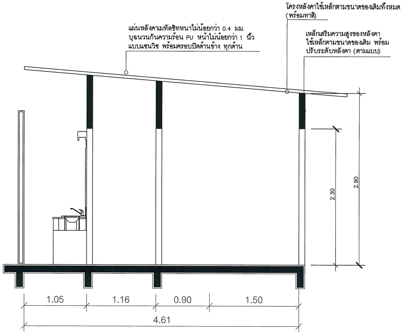
แบบเสริมเหล็กรับหลังคา
