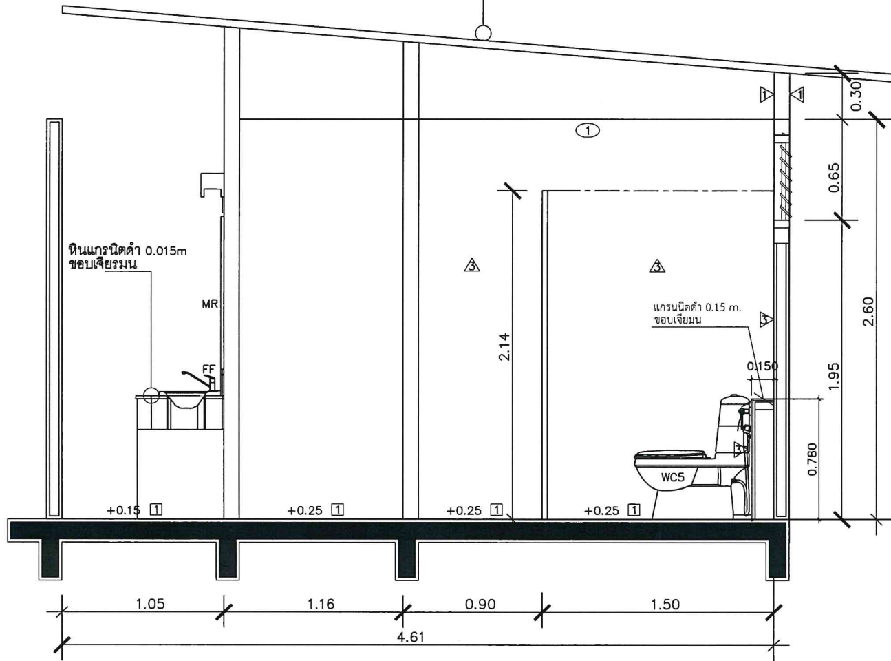
รูปตัด A
